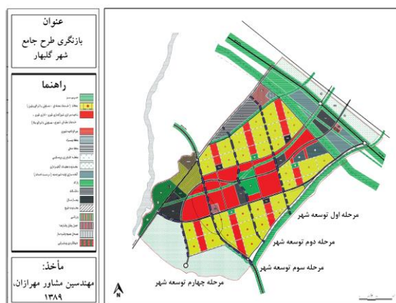
شکل ۳. طرح جامع شهر جدید گلبهار، ۴ مرحله توسعه
